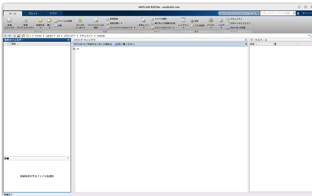
図 4.16: MATLAB
