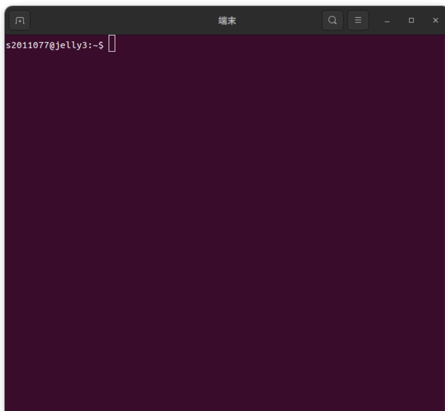
図 1.3: 「端末」の画面
