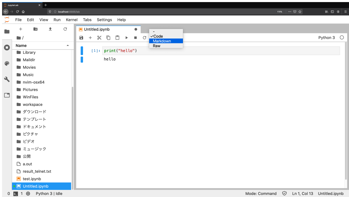
図 4.13: Markdown モード
