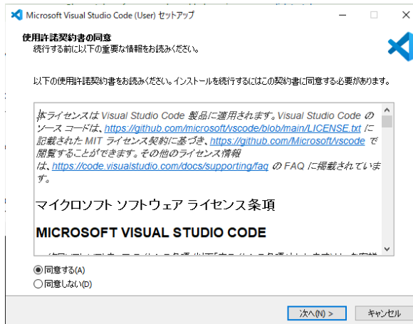
図 2.2: 同意画面
