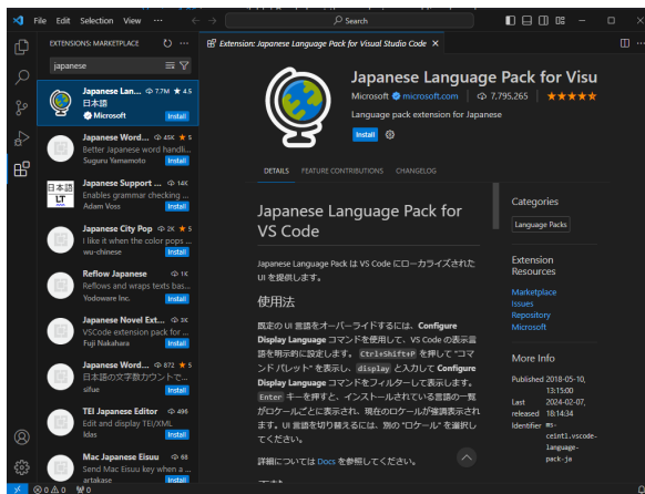
図 2.8: Japanese Language Pack のインストール画面
