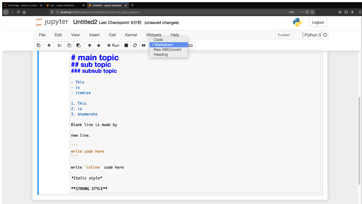
図 4.7: セルのタイプを Markdown にする
