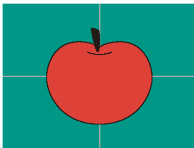
図 3.6: 画像の挿入
