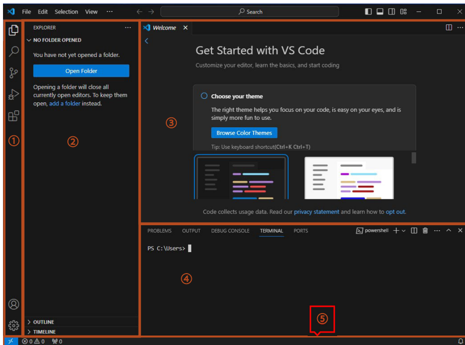
図 2.11: 実際の画面
