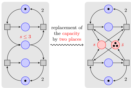
図 3.11: http://www.texample.net/tikz/examples/nodetutorial/
