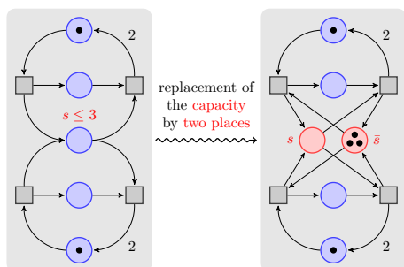
図 6.11: http://www.texample.net/tikz/examples/nodetutorial/
