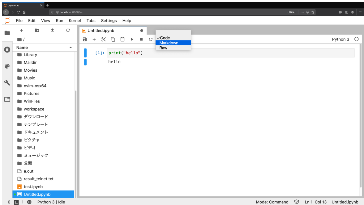
図 7.13: Markdown モード
