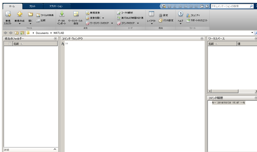
図 7.17: MATLAB
